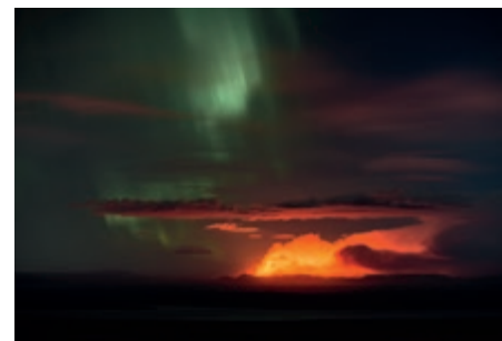
Nordlichter über dem Ausbruch von Holuhraun
